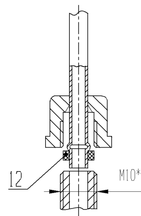
Подсоединение импульсных трубок и трубки запальника
